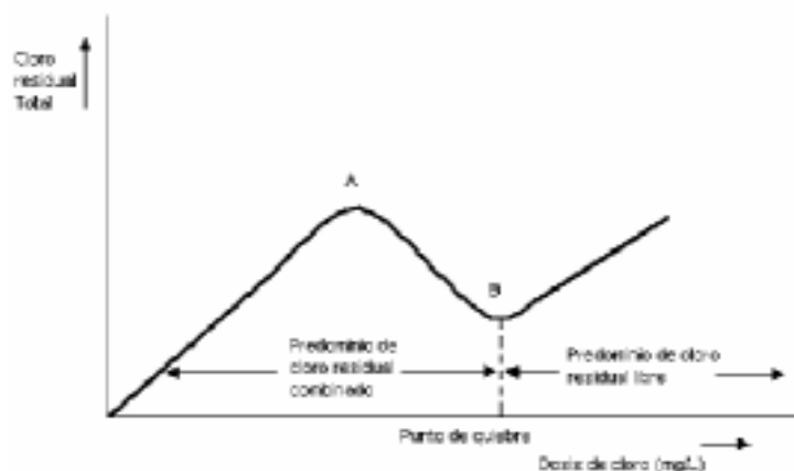
FIGURA C.8.1. Curva de demanda de cloro
